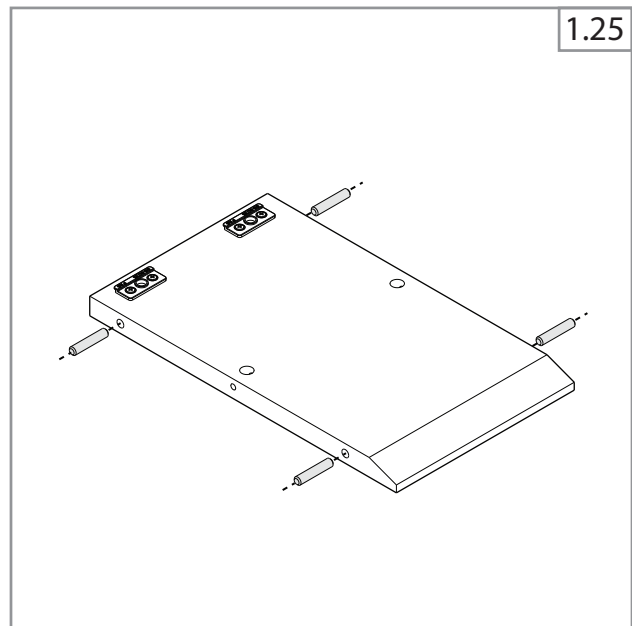
Holzdübel in Einfüllplatten einschlagen Press wooden dowels into filler tops Enfoncer les chevilles en bois dans les plans de jonction
