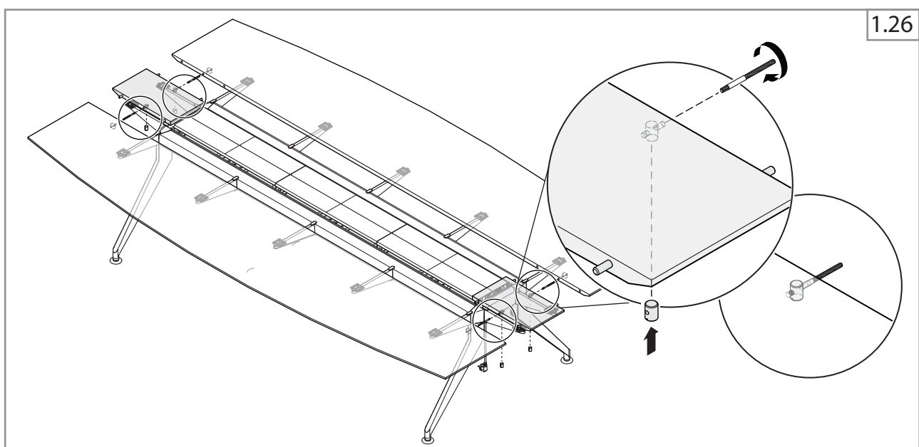
Verbindungsbeschlag in Einfüllplatte eindrücken und Verbindungszapfen festschrauben. Einfüllplatte an erster Hauptplatte ansetzen Push the levelling chock bar into the filler top and tighten the fastening adapter. Join the filler top to the first main top. Enfoncer l'élément de liaison dans le plan de jonction et visser l'adaptateur de fixation. Fixer le plan de jonction sur le premier plateau
